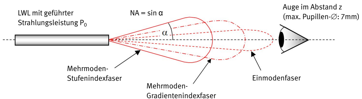
Abb. 1 Strahlprofile nach Austritt aus verschiedenen Fasertypen
